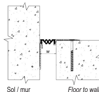
JDH 5.26-040 A avec cornière invisible with invisible side plate
