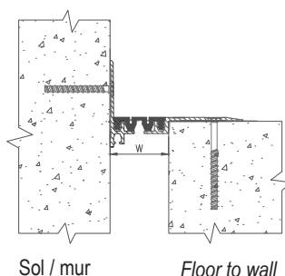
JDH 5.26-050 A avec cornière apparente with visible side plate
