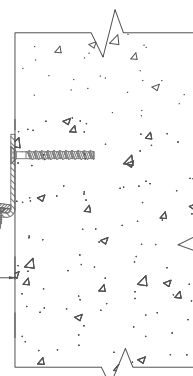
JDH 6.26-050 A avec cornière apparente With visible side plate
