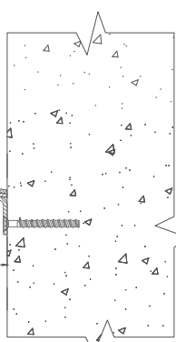
JDH 6.26-050 A avec cornière invisible With invisible side plate
