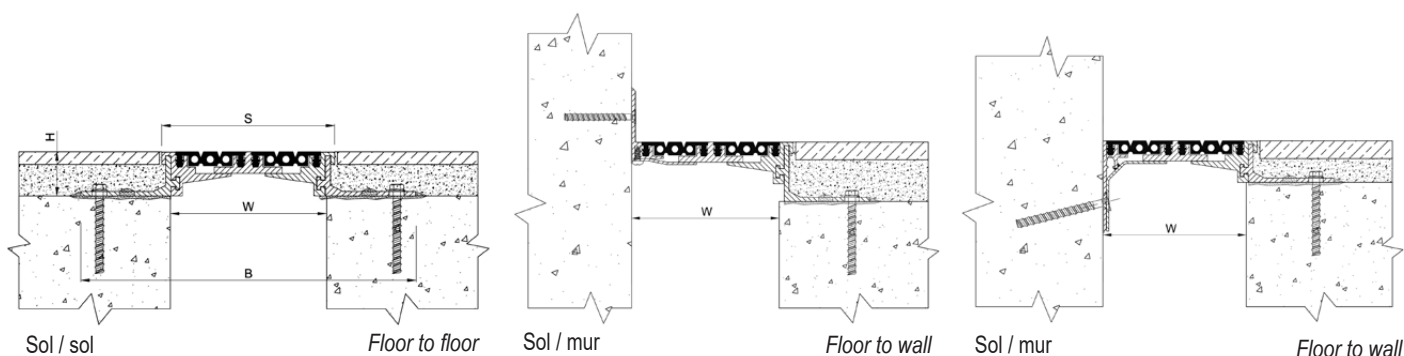
JDH 5.08 A avec cornière apparente With visible side plate
