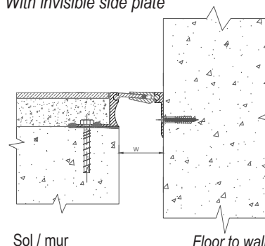
JDH 6.08-050 A avec cornière invisible With invisible side plate
