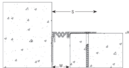
JDH 5.26-040 A (Angle) invisible side part
