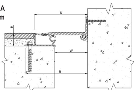
Sol / mur
