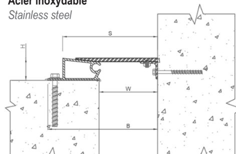
Sol / mur
