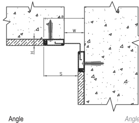
JDV 4.02 A
