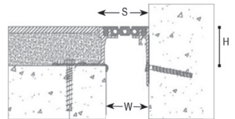
JDH 5.02-050 H50 A con cantonera invisible a partir de la altura 50
