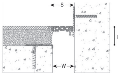
JDH 5.02-050 H50 A con cantonera visible
