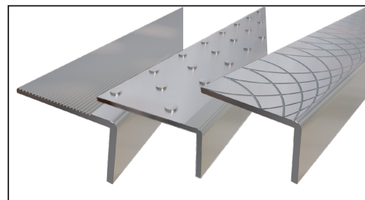
NDM VDi arabesque avec perçage / arabesque NDM VDi with drilling
