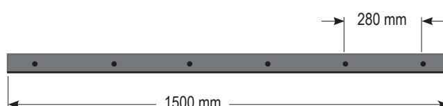
NDM VDi arabesque avec perçage / arabesque NDM VDi with drilling
