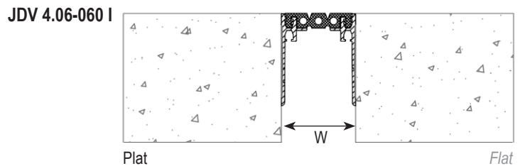
Cornières invisibles collées ou fixées mécaniquement Invisible glued or mechanically fixed aluminium side plates
