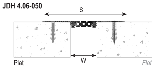
Cornières apparentes fixées mécaniquement Visible mechanically fixed aluminium side plates
