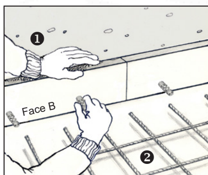
4. Fixer les ressorts d'ancrage en partie basse des bandes VEDAFEU P® Face B selon disposition ci-dessous à droite.
