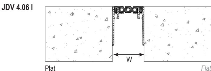
JDV 4.06 I Cornières invisibles collées ou fixées mécaniquement Invisible glued or mechanically fixed aluminium side plates
