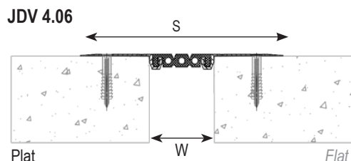
JDV 4.06 Cornières apparentes fixées mécaniquement Visible mechanically fixed aluminium side plates
