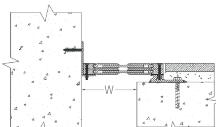
Suelo / pared
