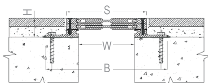
Suelo / suelo
