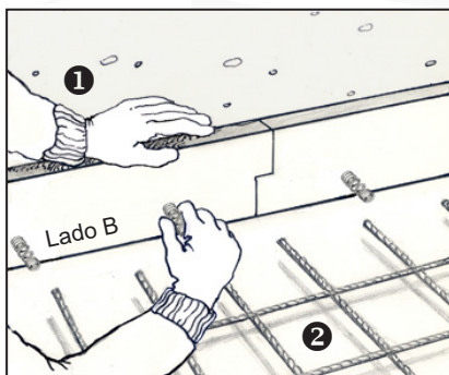
4. Fijar los muelles de anclaje en la parte inferior de las placas VEDAFEU FB® Cara B según la disposición de la derecha.
