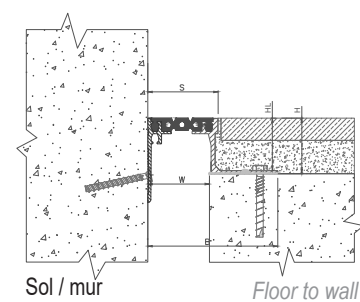
JDH 5.02-060 A cornière invisible
