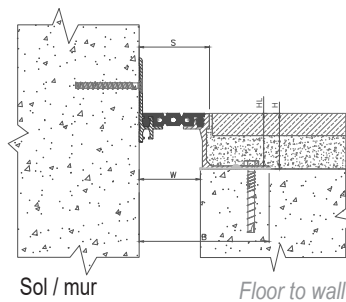
JDH 5.02-060 A cornière apparente
