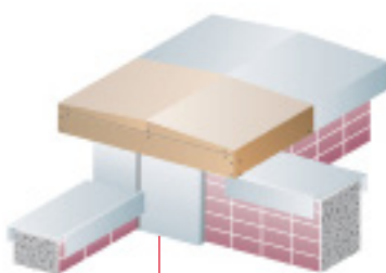
Junta de dilatación vertical versión angular con junta de techo plana
