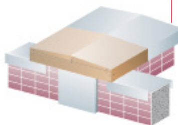
Junta de dilatación vertical con junta de techo plana
