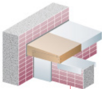
Junta de dilatación vertical versión angular con junta de techo angular
