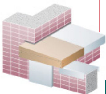
Junta de dilatación vertical con junta de techo angular
