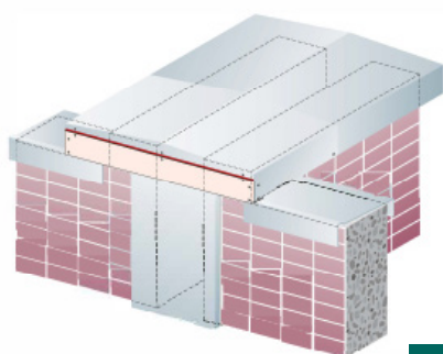
Junta de dilatación vertical con junta de techo angular
